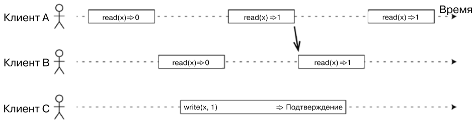
Рис. 9.3. После того как операция чтения вернет новое значение, все последующие операции чтения (для этого и других клиентов) также должны возвращать новое значение
