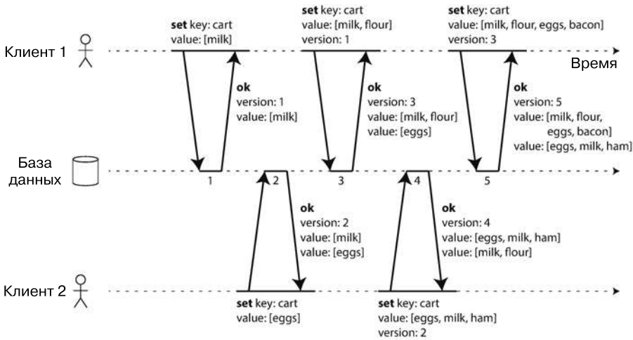
Рис. 5.13. Причинно-следственные зависимости между двумя клиентами, конкурентно редактирующими корзину заказов
